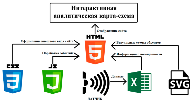
Рис. 1. Концептуальная схема интерактивной карты-схемы
