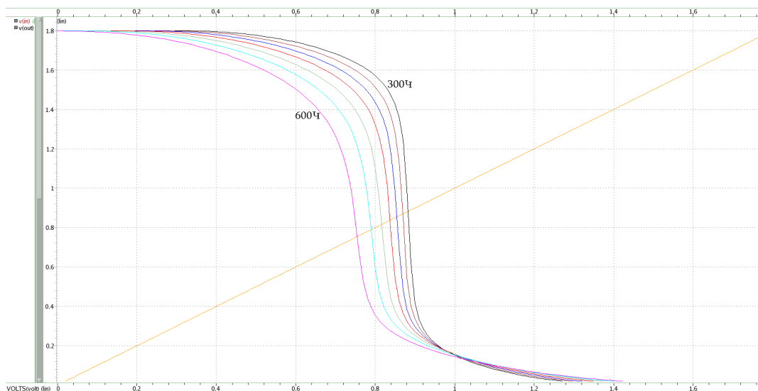
Рис. 2. Температурная зависимость характеристики инвертора
