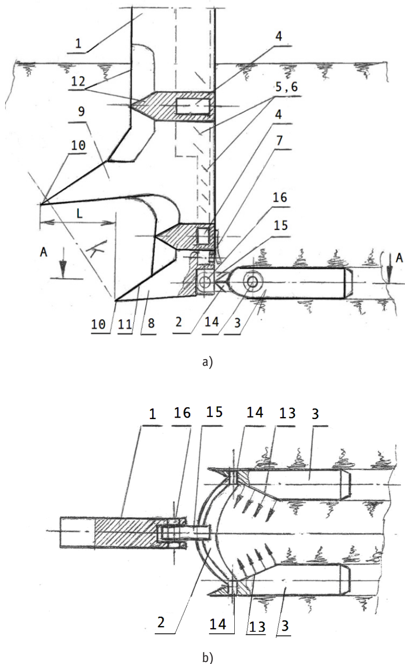
Рис. 1. Схема устройства, вид сбоку (а) и разрез А-А (b): 1 — вертикальный нож; 2 — нижний задний части режущей подковы; 3 — дренары; 4 — полость; 5 — боковые сопла; 6 — узкий щель; 7 — клапан; 8 — нижний долотообразный зуб; 9 — верхний долотообразный зуб; 10 — носок долотообразный зуб; 11 — нижний зуб; 12 — клиновидный зуб; 13 — усечение дренары; 14 — шарнир; 15 — тяга; 16 — шарнир
