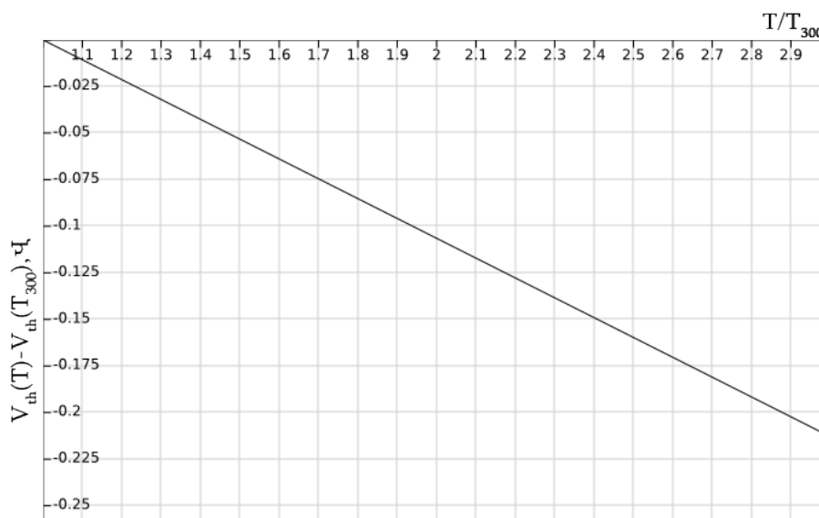
Рис. 1. Зависимость порогового напряжения от температуры
